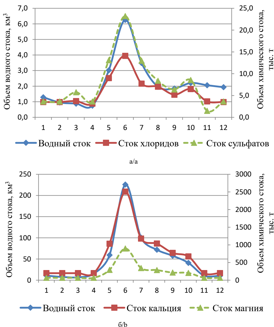
Рис. 2. Внутригодовое изменение водного и химического стока арктических рек при смещении максимумов кривых (а – р. Печора; б – р. Яна) / Fig. 2. Intra-annual change in the water flow and chemical runoff of Arctic rivers with a shift in the maxima of the curves (a - Pechora river; b - Yana river)
